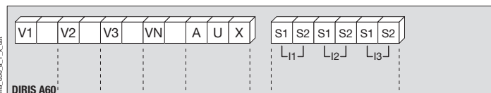
DIRIS A60
