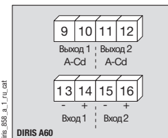
Модуль с 2 входами / 2 выходами
