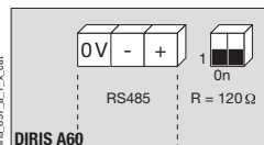
Коммуникационный модуль
