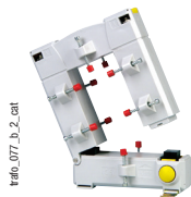
Трансформаторы тока с разъемным сердечником
