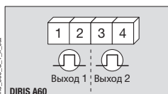
Модуль импульсных выходов
